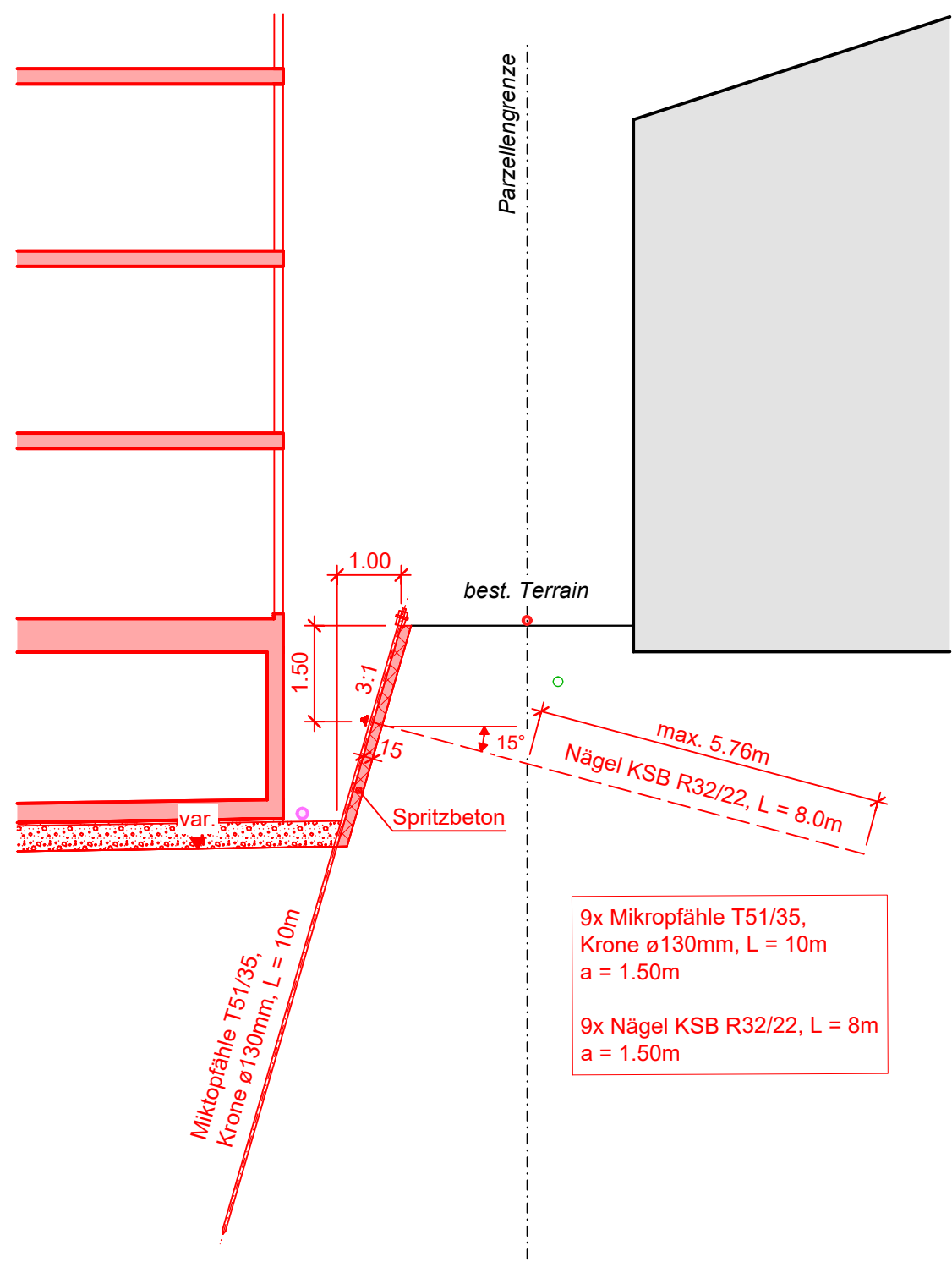
Schemaschnitt 1:50 Bodenaufbau Baugrube, mit Dämmung
