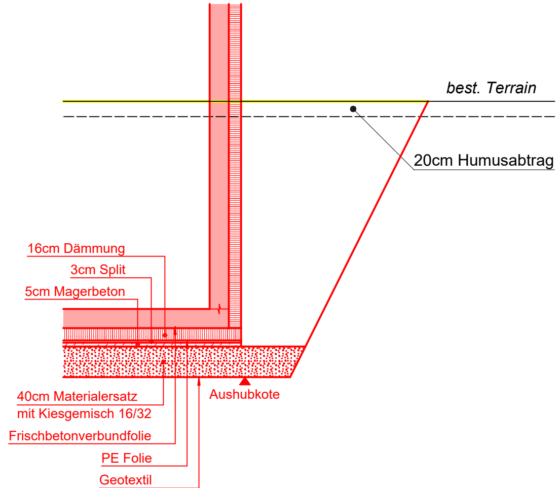
Schemaschnitt 1:50 Bodenaufbau Baugrube, mit Dämmung
