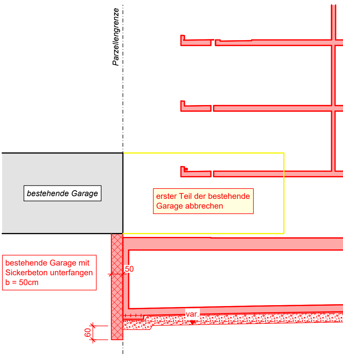
Schnitt C 1:100
