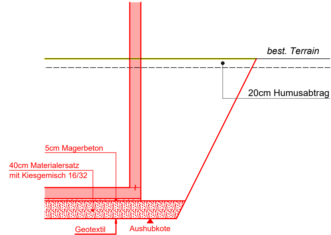
Schemaschnitt 1:50 Bodenaufbau Baugrube, ohne Dämmung
